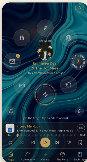
Сцена
