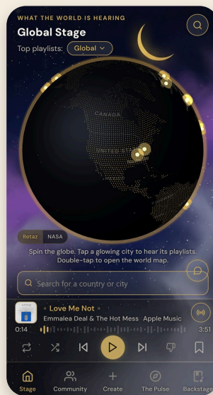
Глобальная сцена
