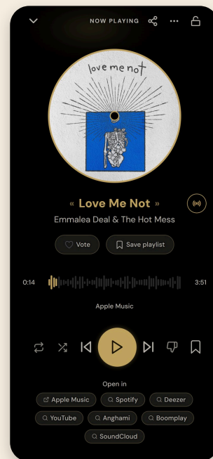
Сейчас играет
